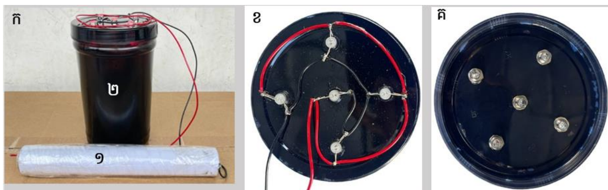
រូបភាពទី៣៖ ឧបករណ៍ពិសោធន៍ផលិតរួច
